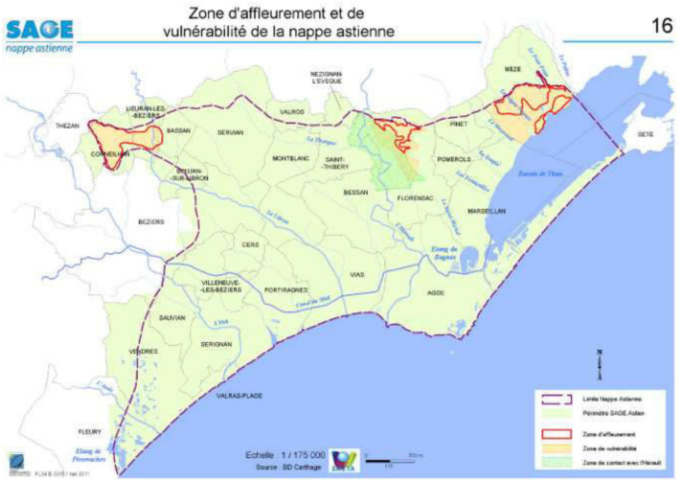
Figure 7 : Zones d'affleurement et de vulnérabilité de la nappe astienne
