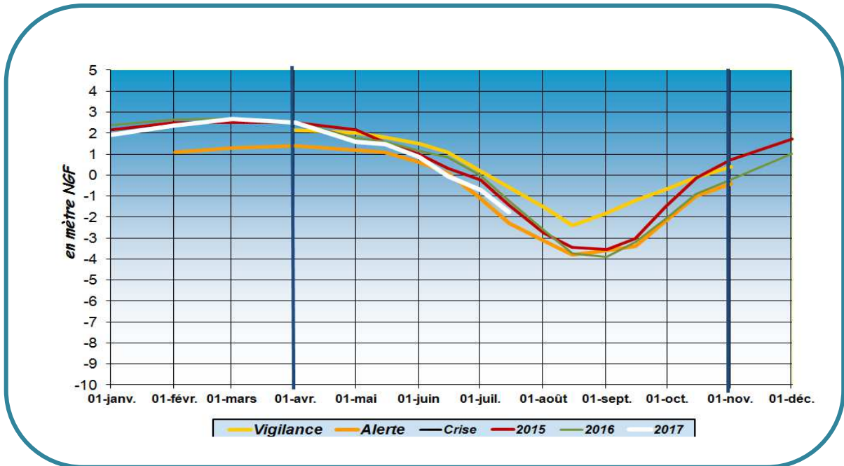
Évolution du niveau de la nappe à Sérignan - n°2
